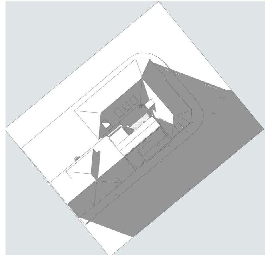
Soldiagram 23 juni kl 20 - planlagt
