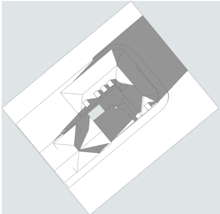
Soldiagram 21 mars (vintertid) kl 15 - eksisterende
